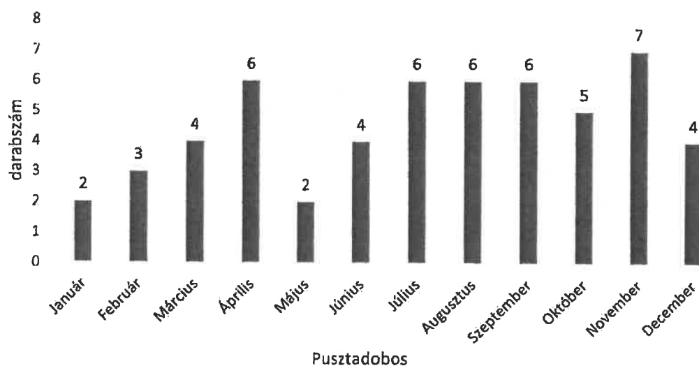
Szennyvíz dugulások alakulása 2018.
